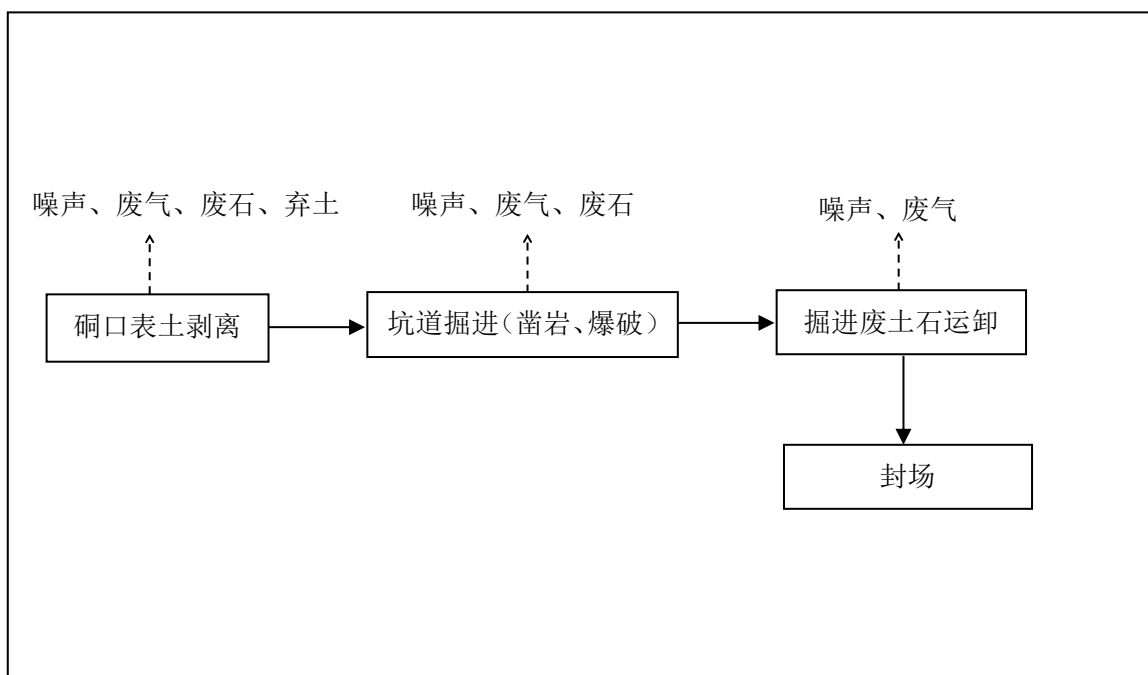
图 5-1 坑探施工工艺流程及产污环节图
