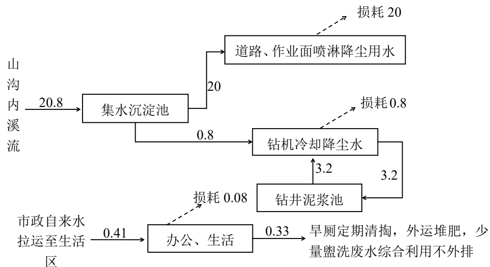
图 1-2 水平衡图 m 3 /d
