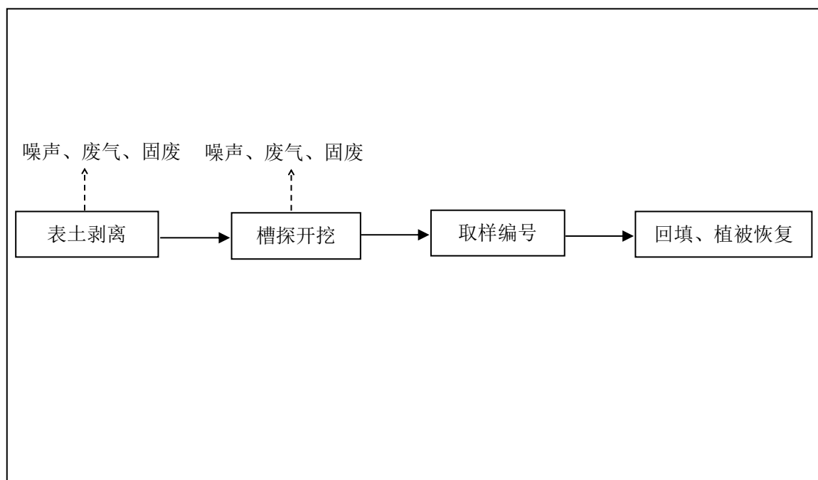
图5-3 槽探施工工艺流程及产污环节图
