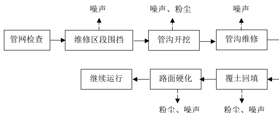
图 5-5 污水收集管网事故检修中工艺流程及污染环节图
