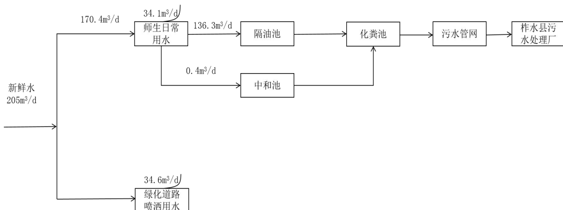
图 1 水平衡图
